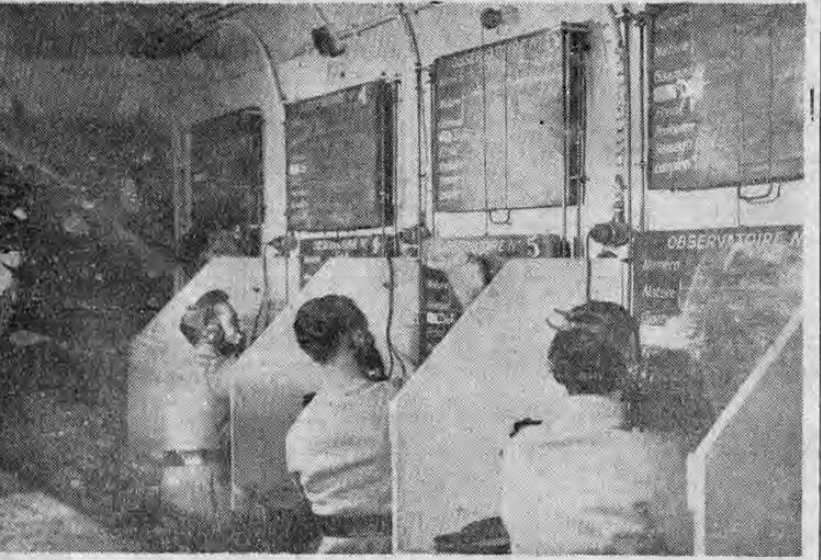
Un puesto de central telefónica de la artillería a 15 metros bajo la superficie del suelo en la línea Maginot; los soldados telefonistas están conectando los puestos de escucha en la línea más avanzada con los comandantes de baterías que son guiados en su tiro por los observadores adelantados que están a centenares de metros del blanco en que explotan las granadas y ven sus efectos y dirigen los tiros.
